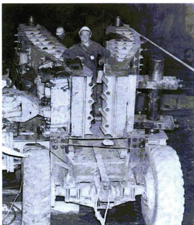
Foto lewej: Obrotowa kruszarka - 02 kwietnia 1973
